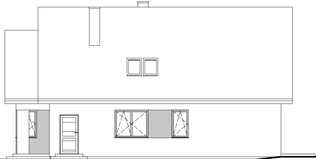
ELEWACJA BOCZNA PRAWA
